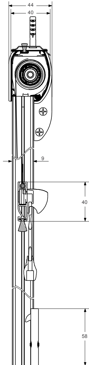
SEZ. VERTICALE
