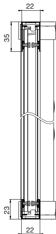
SEZ. VERTICALE
