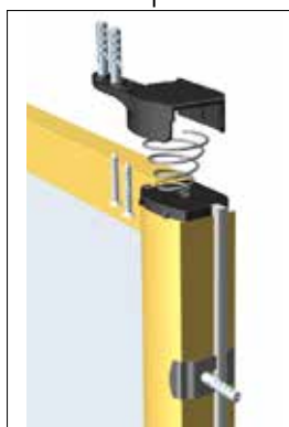
Fissaggio con aletta
